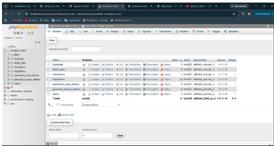
(Screenshot: Halaman phpMyAdmin menunjukkan daftar tabel dari database bengkel_motor)
